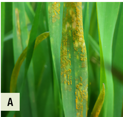
1.kép A sárgarozsda (A) és vöröszsda (B) erős fertőzése búzálevélen
